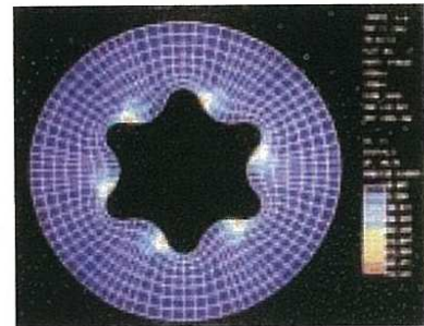
【トルクスの応力分布】
