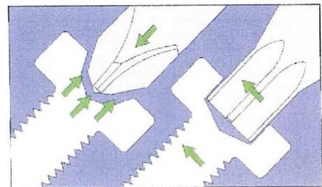
【トルクスの応力分布】
