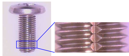
”フィットロック加工” (緩み止め)
